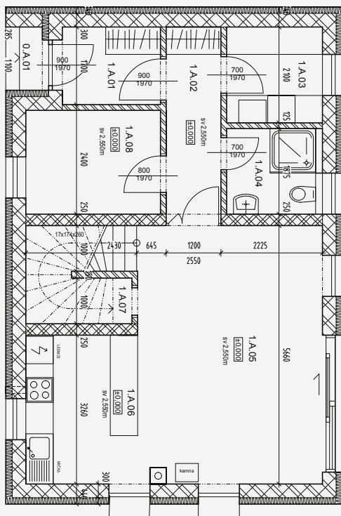
1. NP
