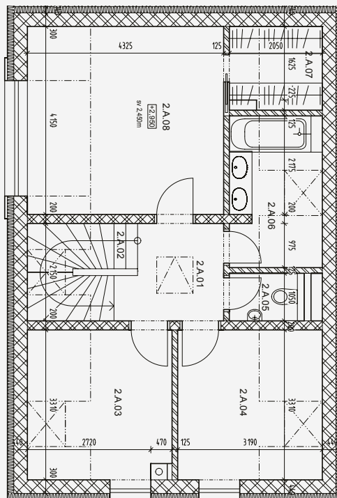
2. NP
